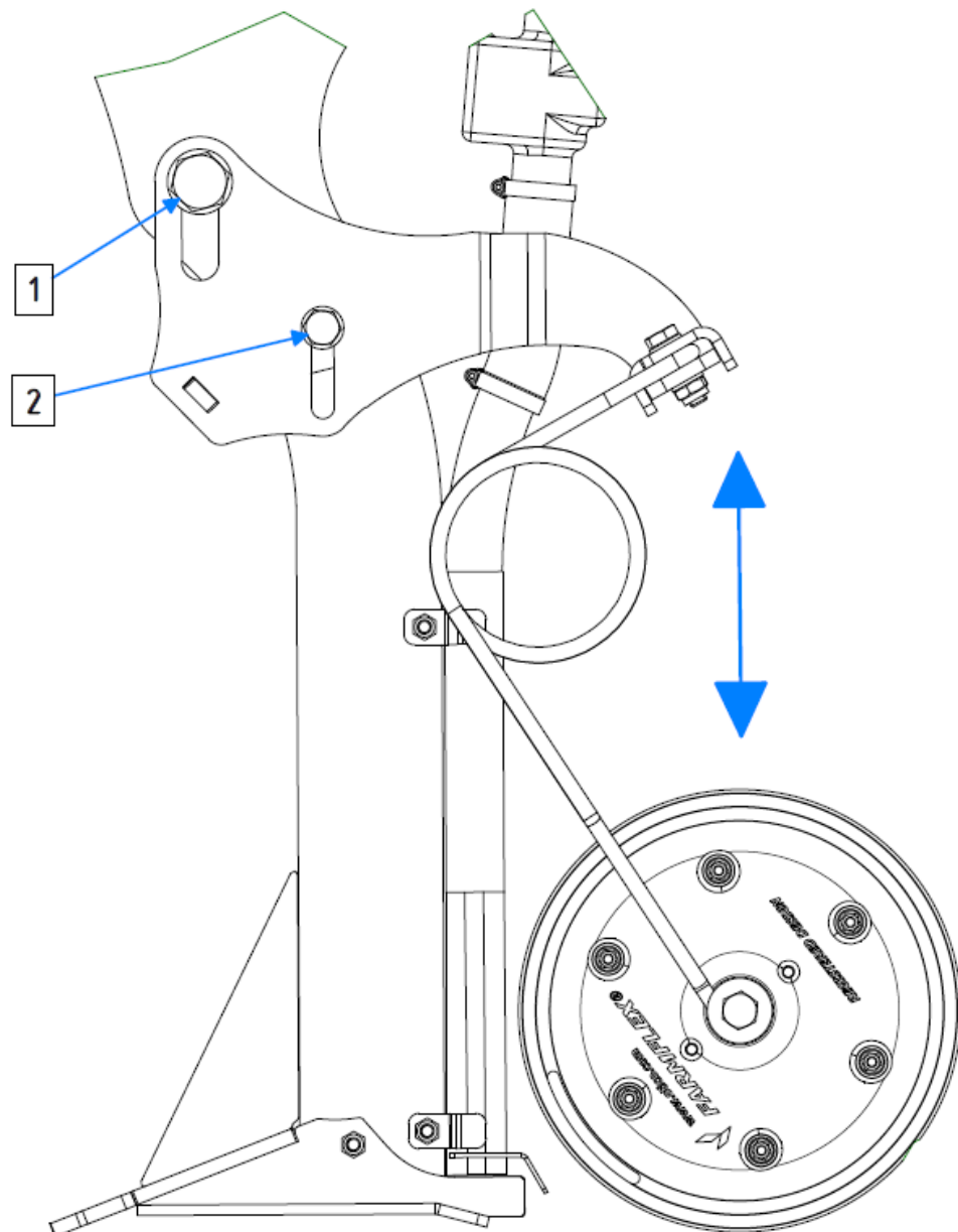
Abb. 46. Einstellen des Rapsrads
