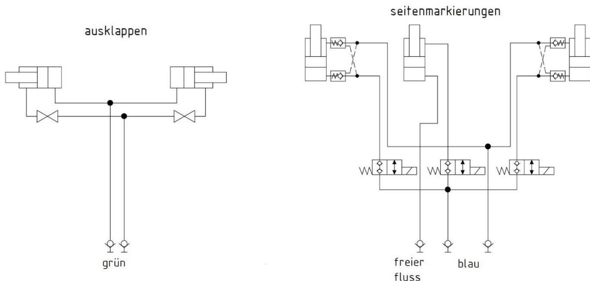
Abb. 17. Hydraulikschema
