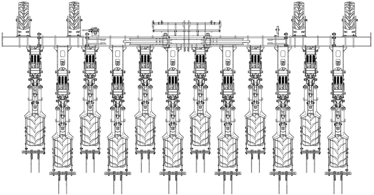
Abb. 43. Abstand 12x45 cm für PS 600
