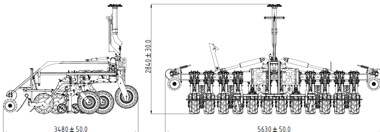
Abb. 9. Außenmaße PS 450 – Betrieb
