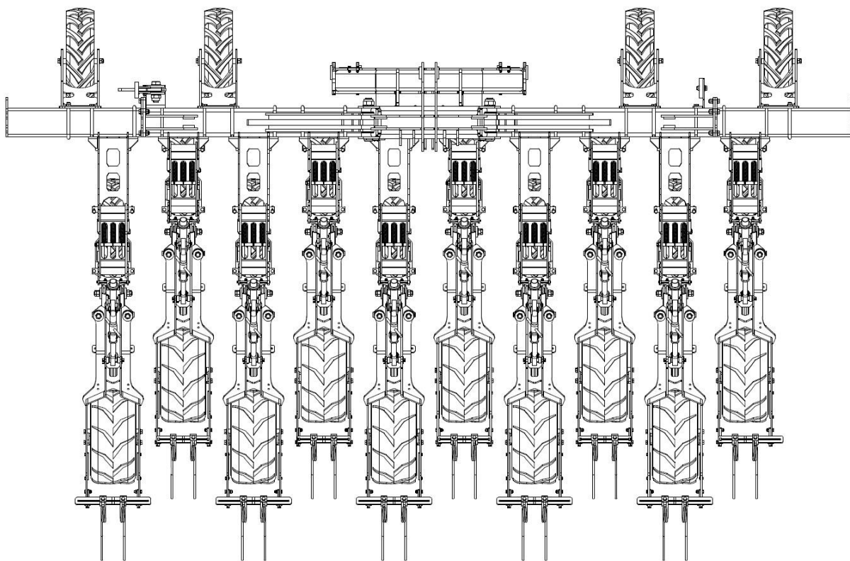
Abb. 39. Abstand 10x40 cm für PS 400
