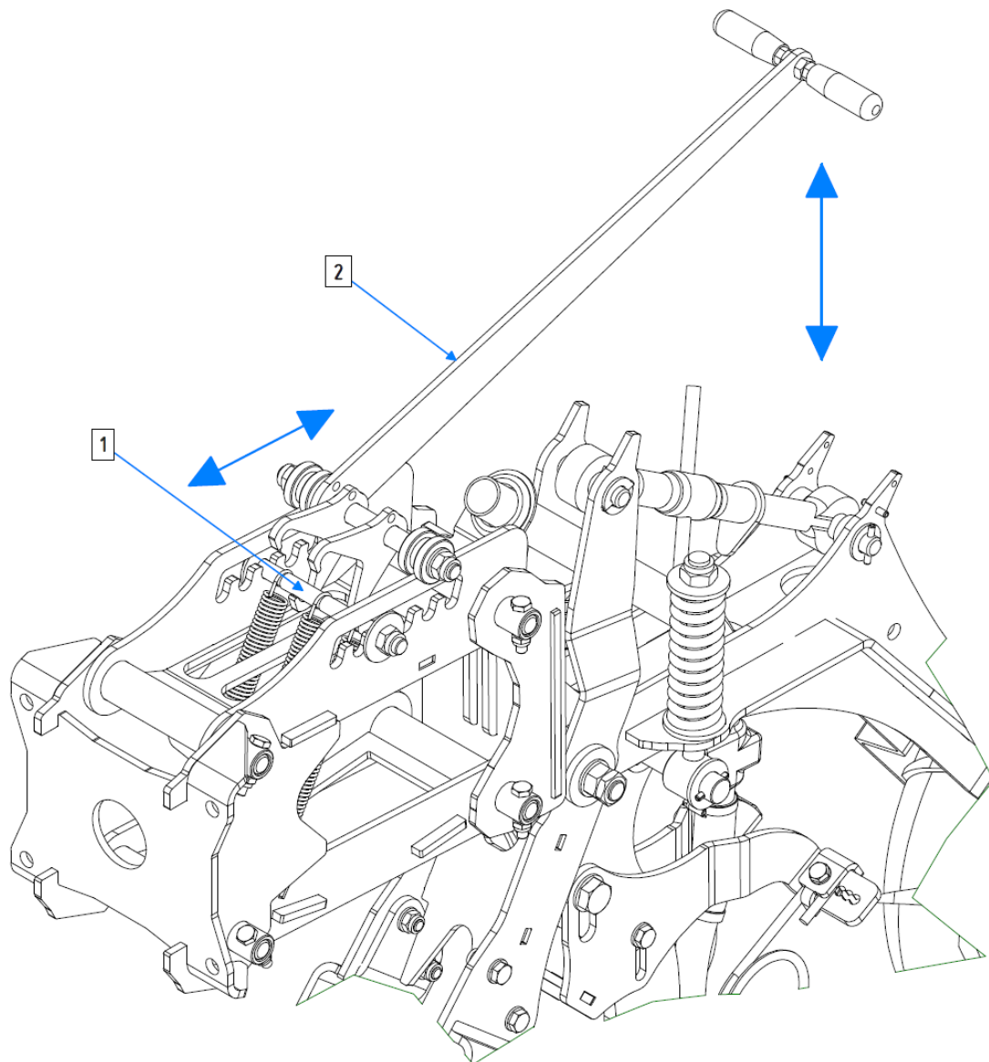
Abb. 45. Einstellung des Drucks im Arbeitsabchnitt
