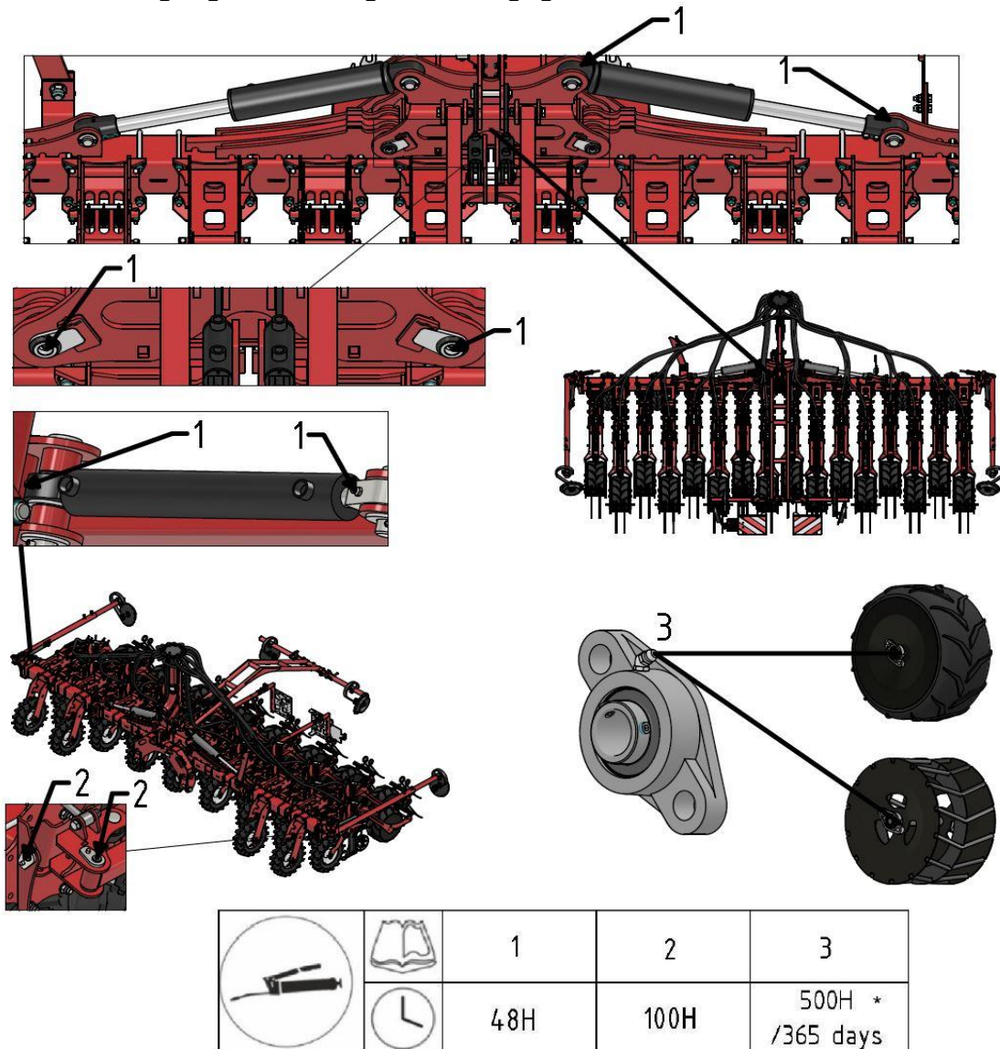
Abb. 27. Schmierstellen
