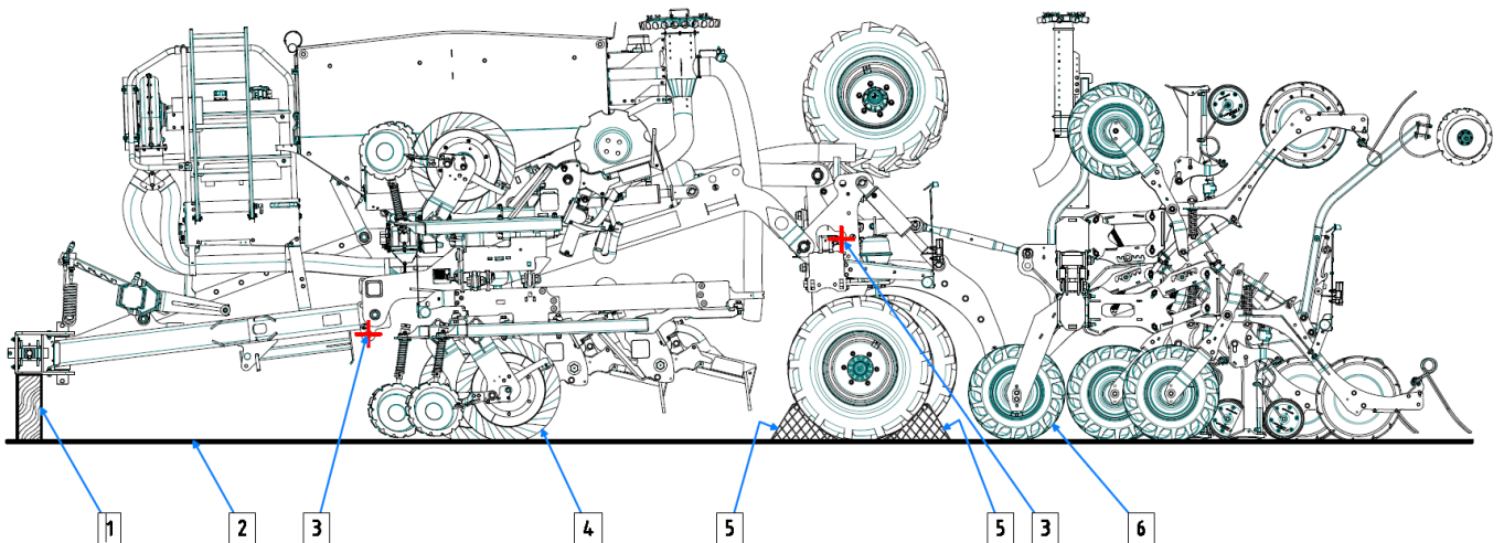
Abb. 52. Maschinensicherungspunkte auf dem Transportmittel
