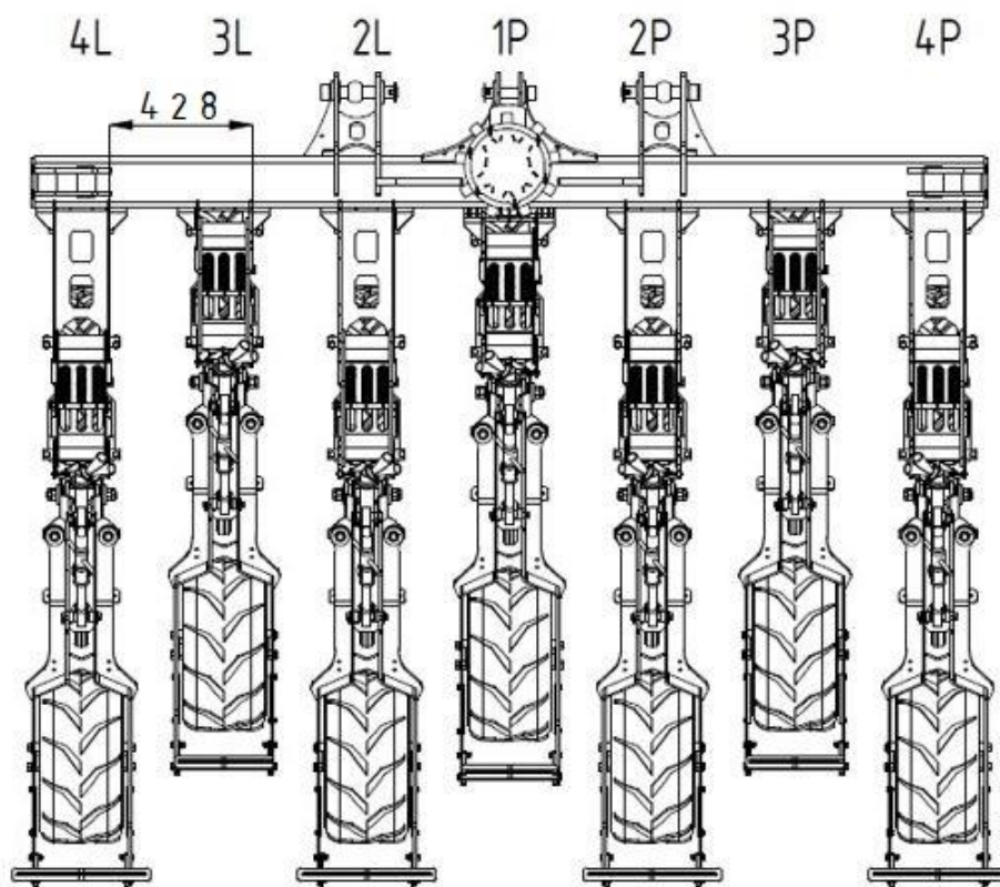
Abb. 25. Abstand 7 x 42,8
