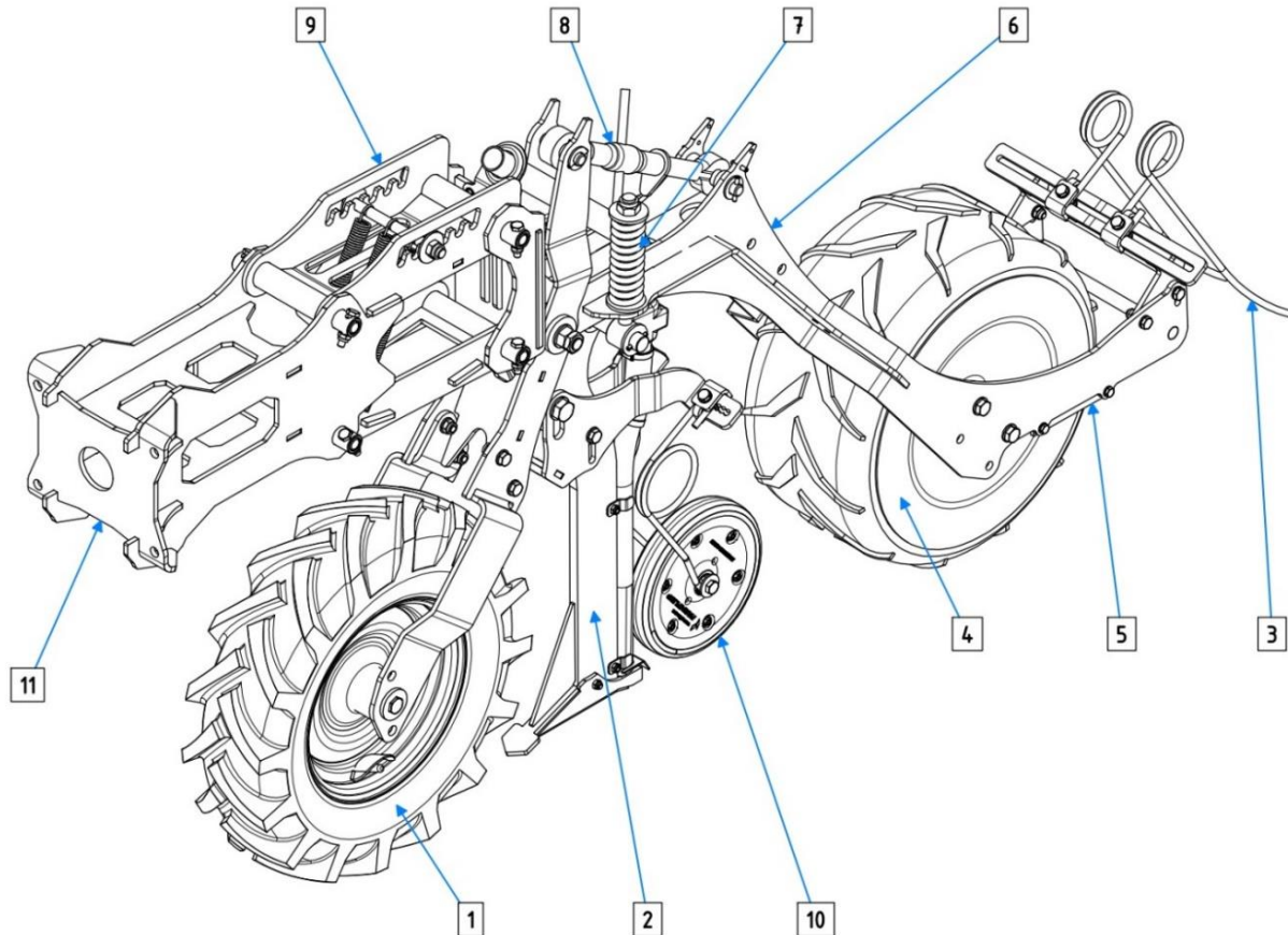
Abb. 29. Arbeitsabschnitt PS mit langer Befestigung (Beispiel mit einer Verdichtungsrolle aus Gummi).
