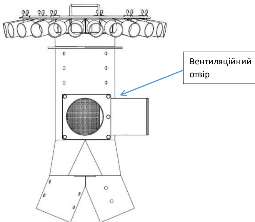
Мал. 102 Головка розподільника насіння.
