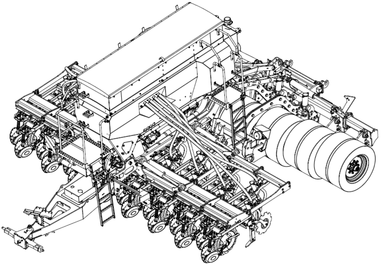
Мал. 94 Вигляд машини ST600 в робочому положенні
