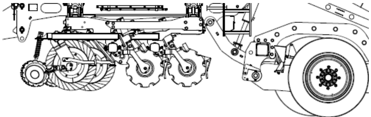
Мал. 101 Спосіб регулювання притискання дисків
