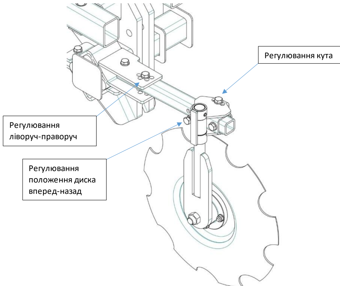
Мал. 100 Спосіб регулювання загібально-замикаючого диска
