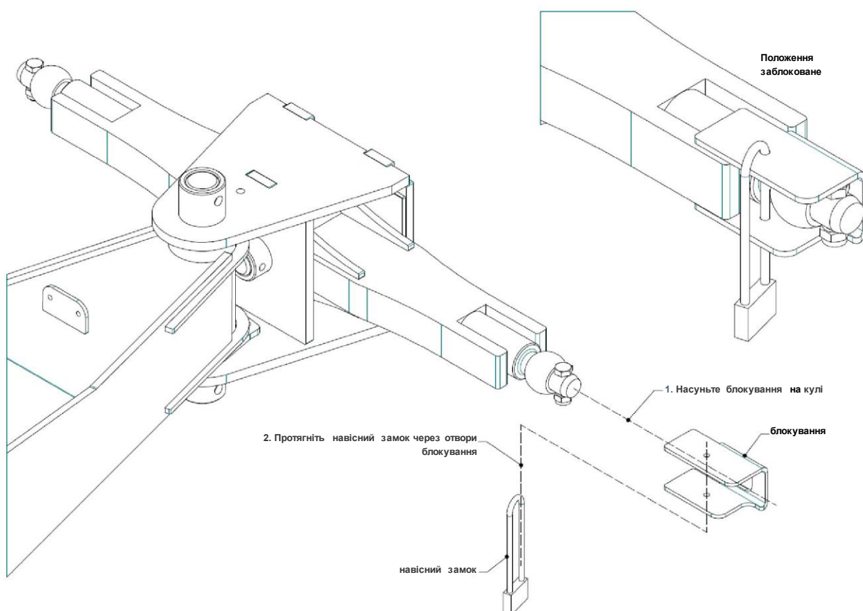
Мал. 104 Блокування зчіпки
