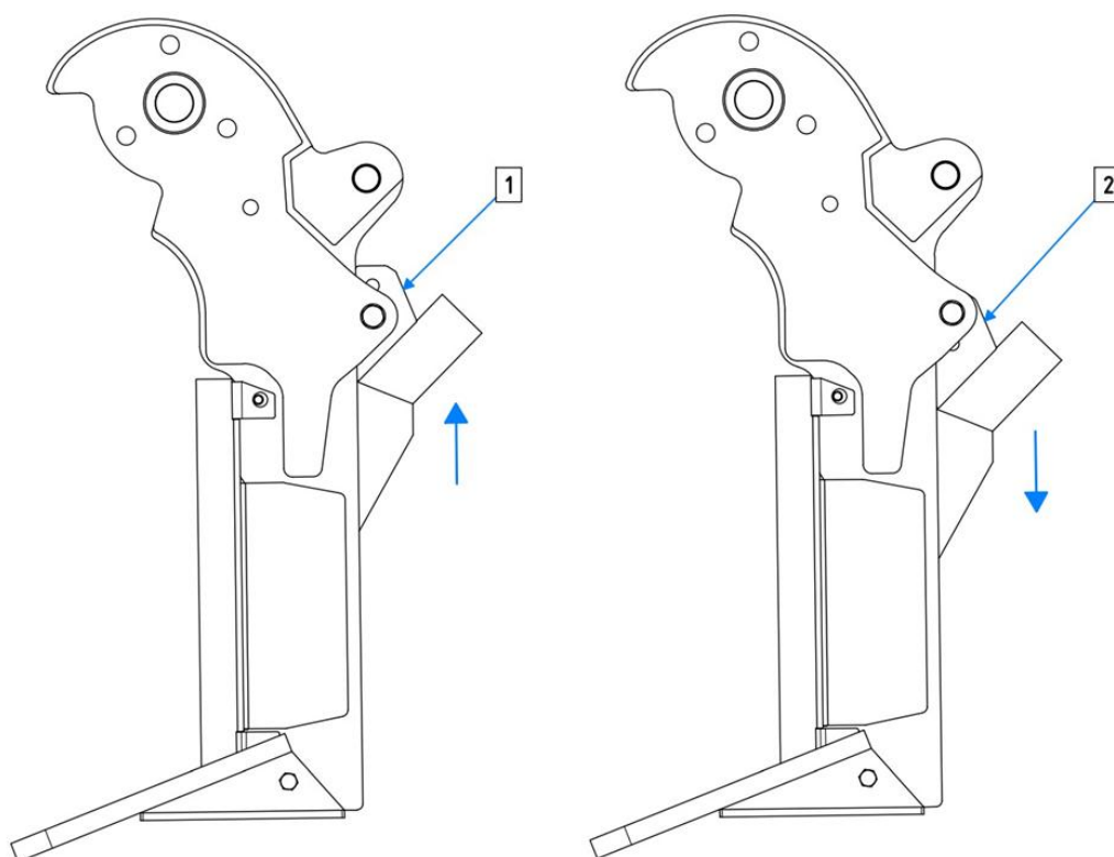
Мал. 96 Регулювання глибини внесення добрив
