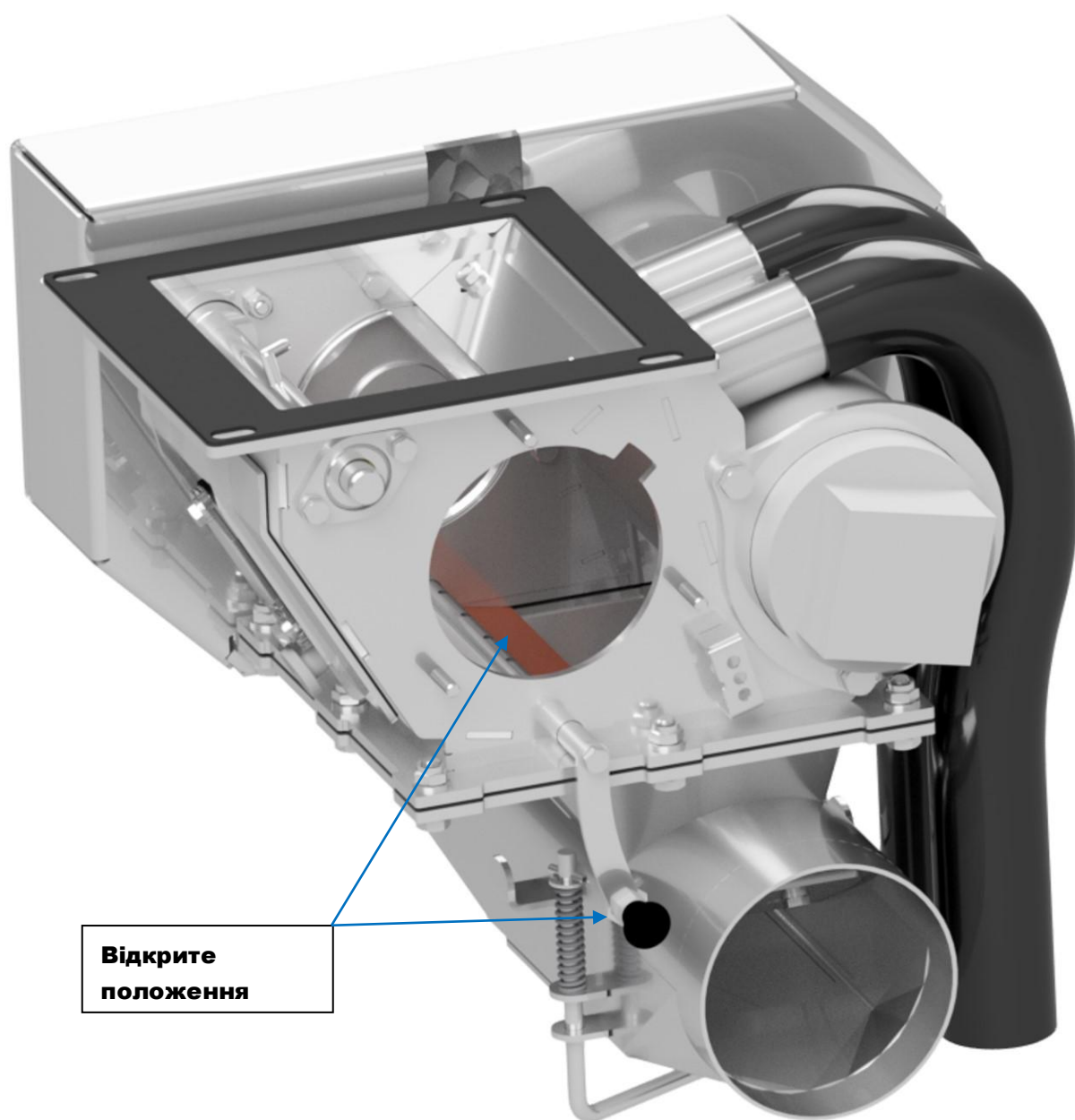
Мал. 79 Скребок у відкритому положенні
