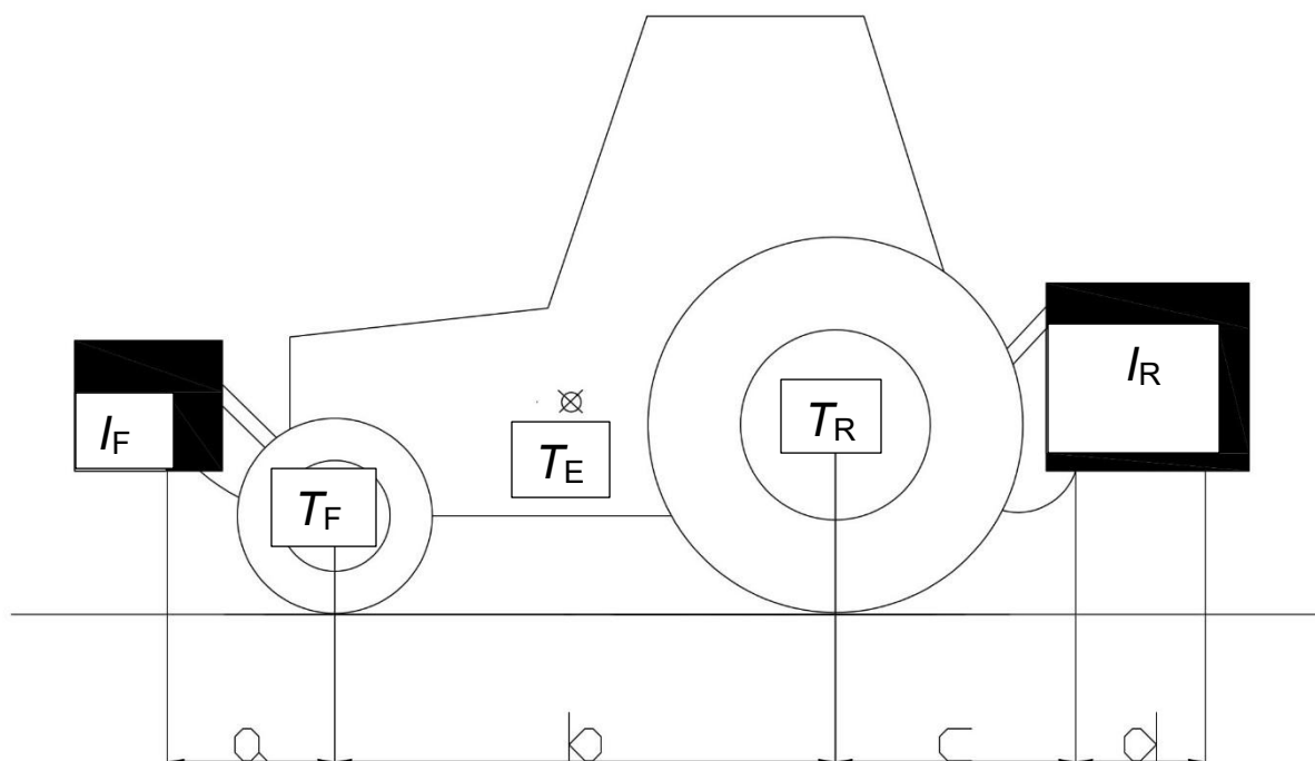
Мал. 10 Схема для розрахунку навантаження
