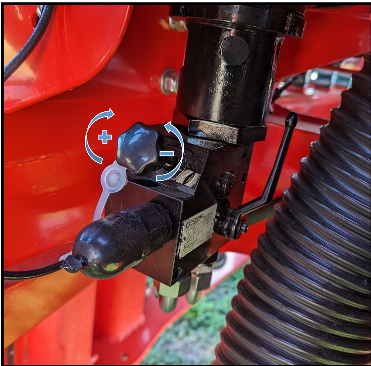
Мал. 74 Спосіб регулювання
