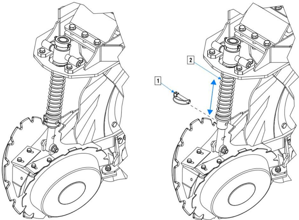
Мал. 97 Спосіб регулювання притискання дисків
