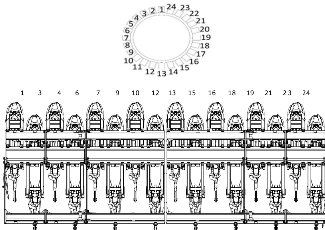
Мал. 68 Схема розташування шлангів ST600 16 рамок
