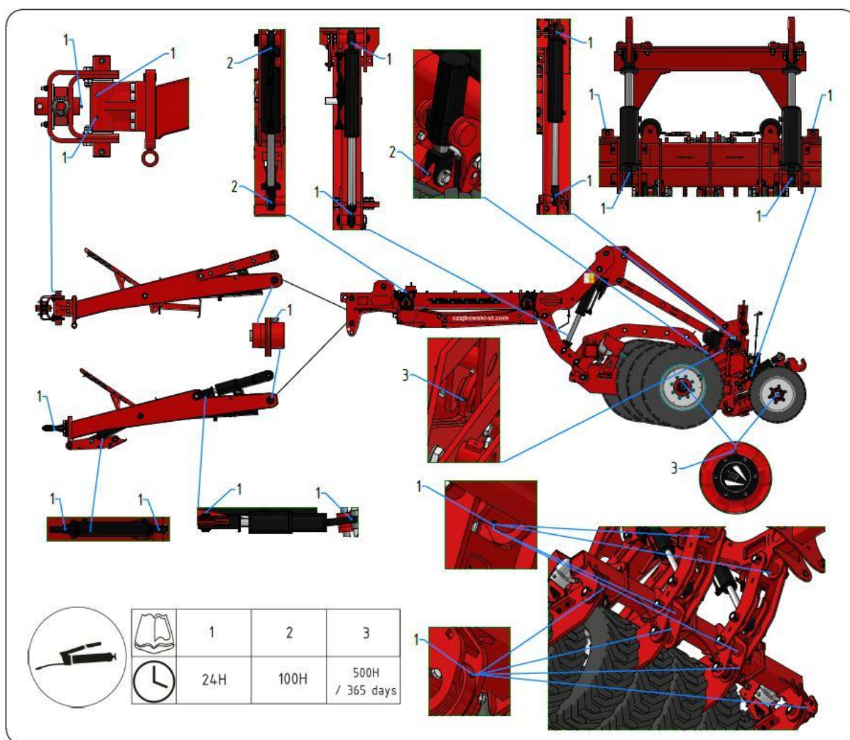
Мал.80. Точки змащування ST
