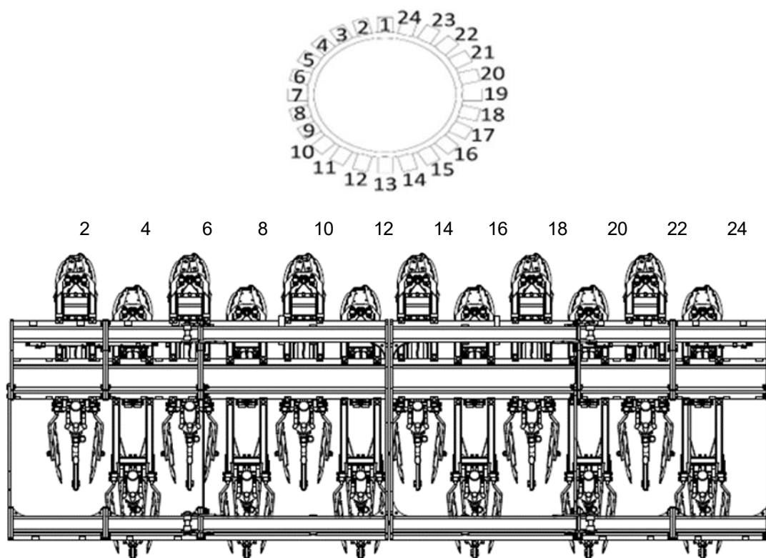
Мал. 69 Схема розташування шлангів ST600 12 рамок
