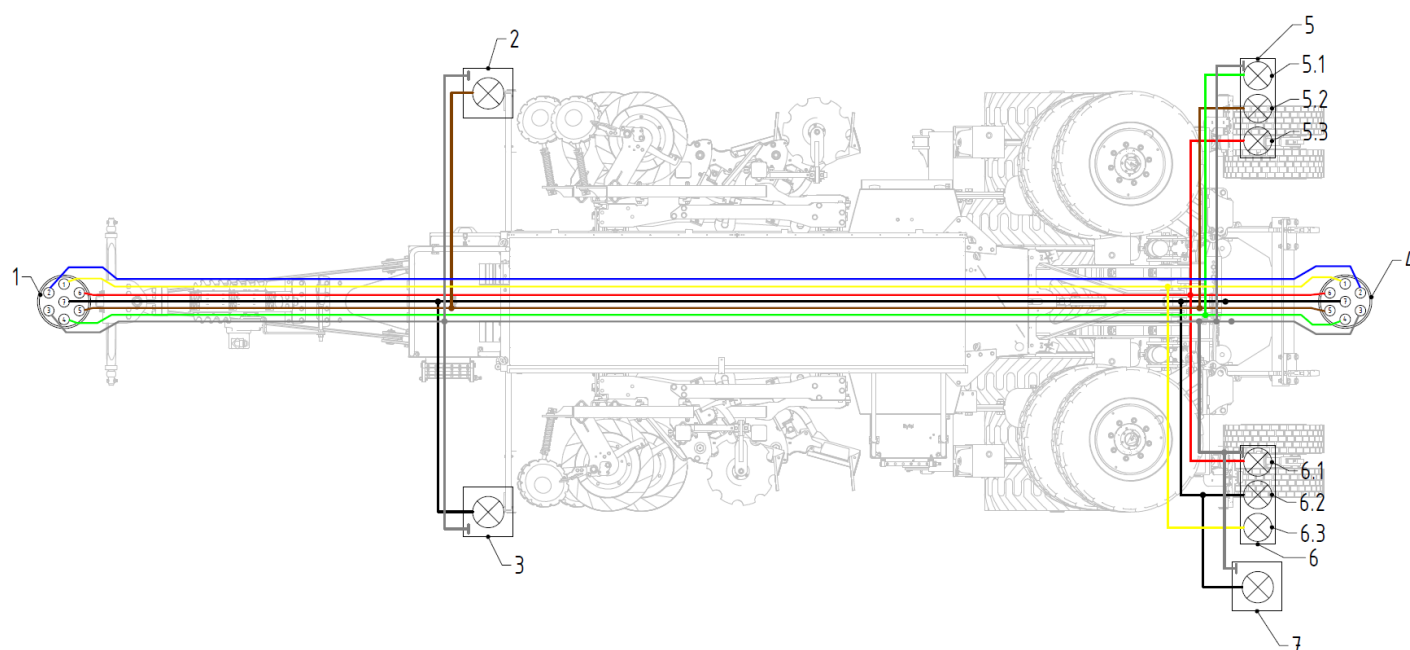
Мал. 55 Схема електричної системи освітлення.
