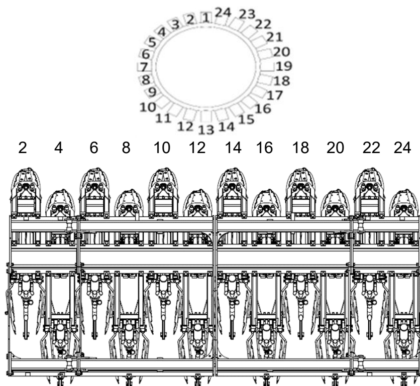
Мал. 71 Схема розташування шлангів ST450 і ST400 12 рамок
