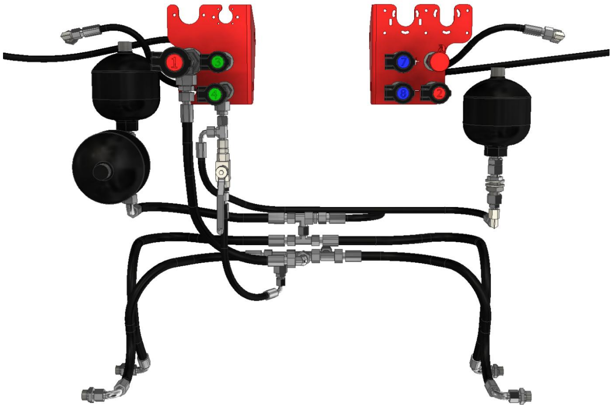
Мал. 73 Задня частина машини CZAJKOWSKI ST
