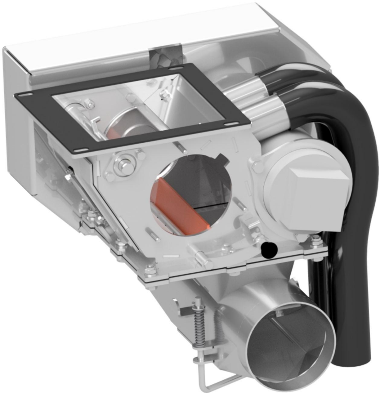
Мал. 78 Скребок у закритому положенні
