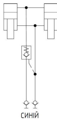
Мал. 46 Принципова схема системи гідравлічної амортизації в ST
