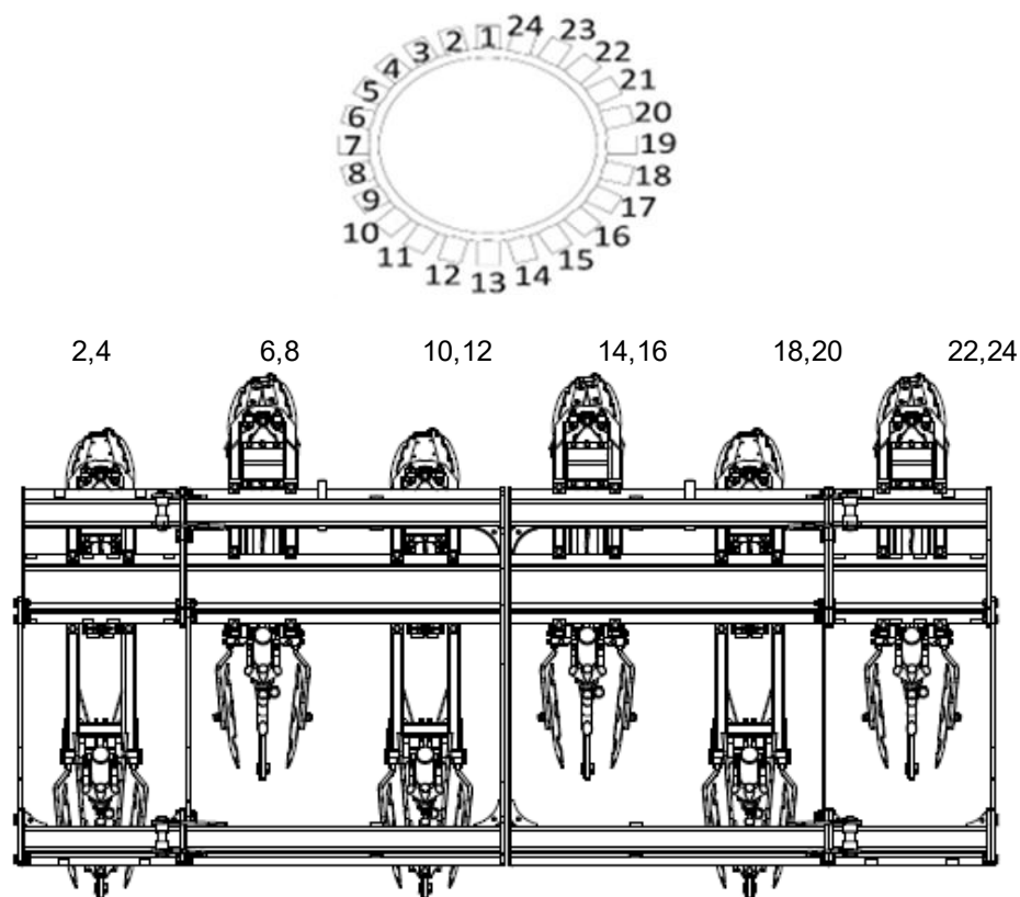
Мал. 71 Схема розташування шлангів ST400/ ST450 6 рамок
