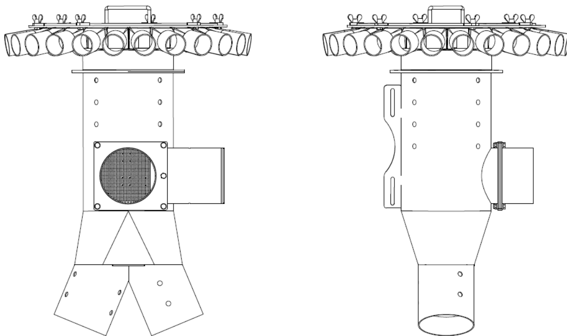
Мал. 77 Головка розподільника насіння
