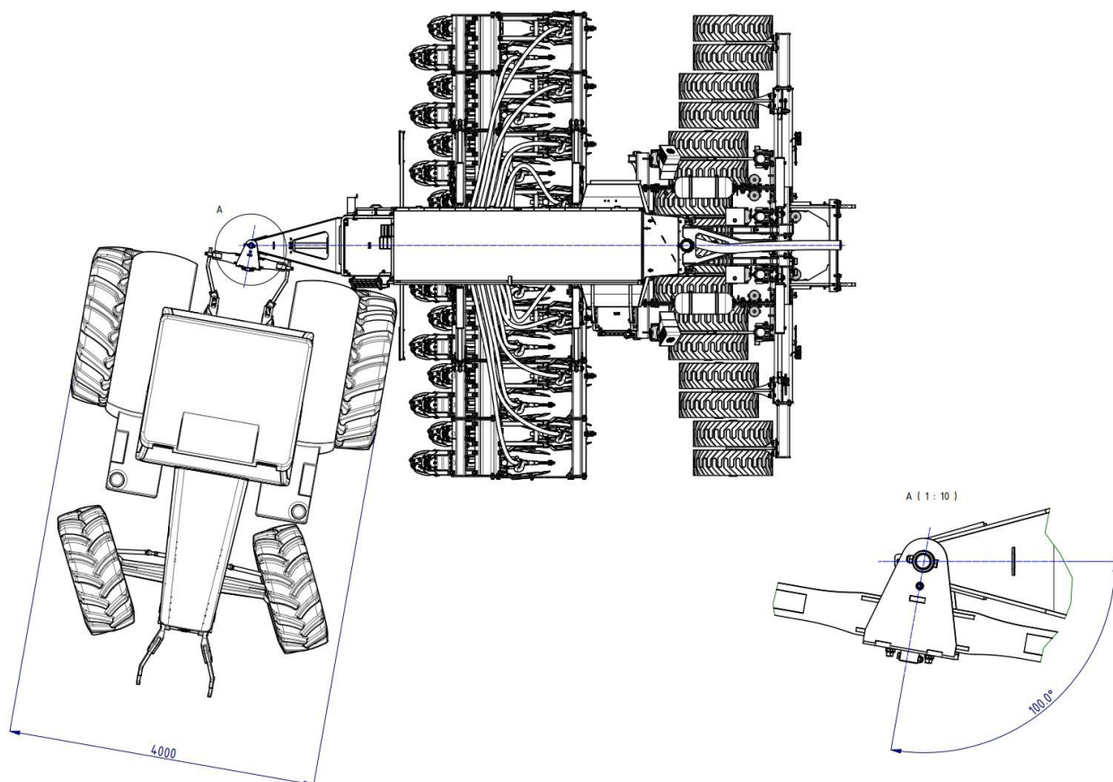
Мал. 105 Максимальна ширина здвоєних коліс трактора.
