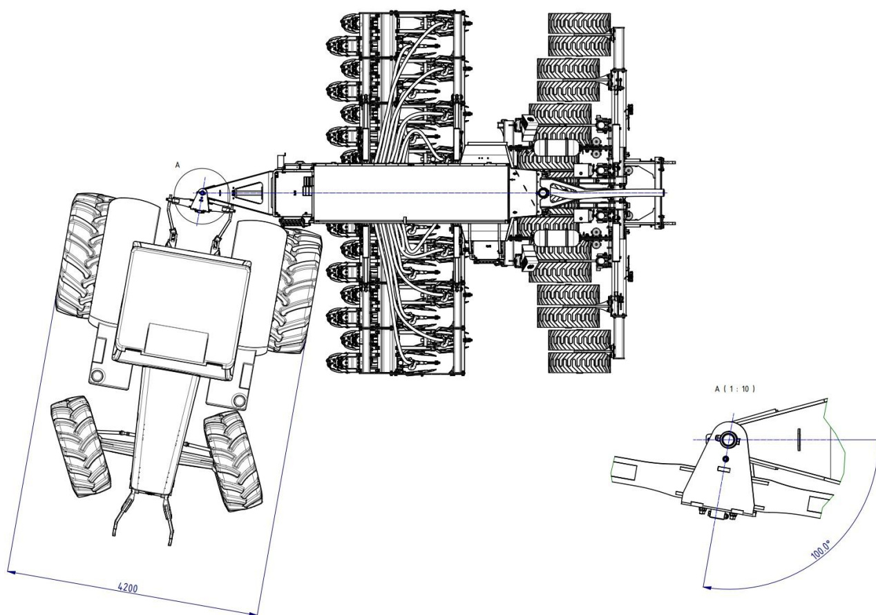
Мал. 106 Максимальна ширина здвоєних коліс трактора зі знятим профілем габаритної дошки
