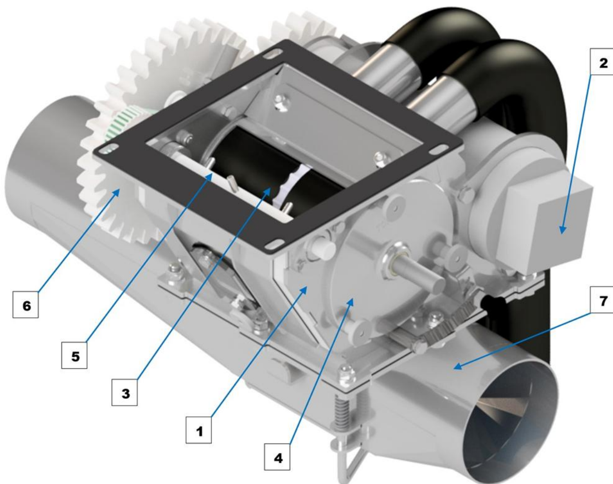
Мал. 81 Висівний апарат.
