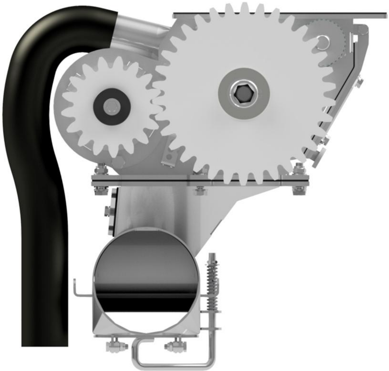
Мал. 84 Зубчасті шестерні висівного апарату.
