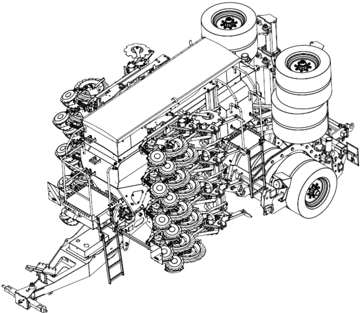
Мал. 92 Вигляд машини ST600 в транспортному положенні
