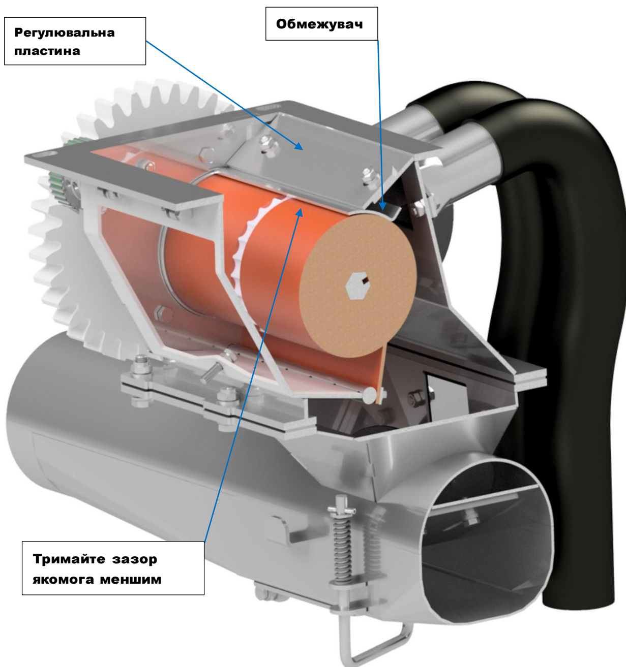
Мал. 87 Регулювання обмежувача.
