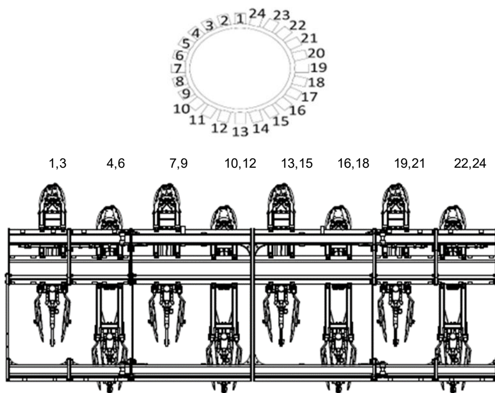
Мал. 70 Схема розташування шлангів ST600 8 рамок
