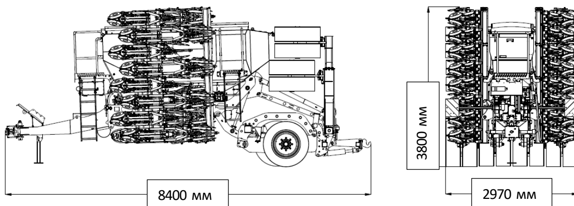
Мал. 5 Габаритні розміри 6-метрової машини без надставки.
