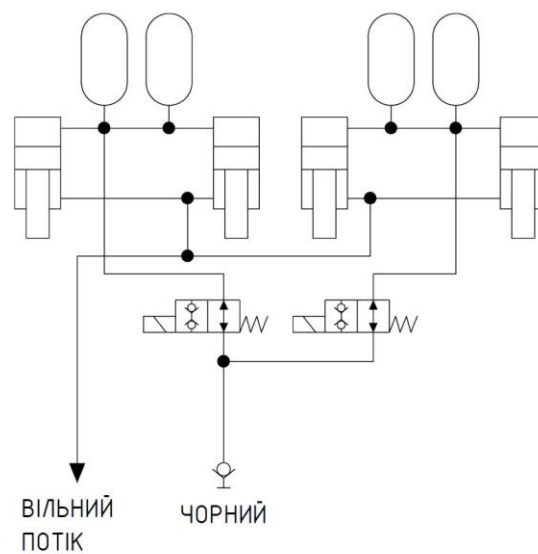
Мал. 46 Принципова схема системи гідравлічної амортизації в ST
