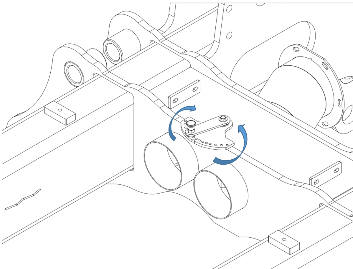
Мал. 103 Елемент керування повітрям.
